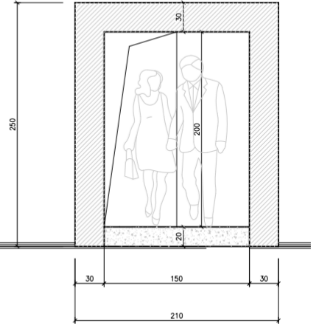
חתך 2-2 1:25
